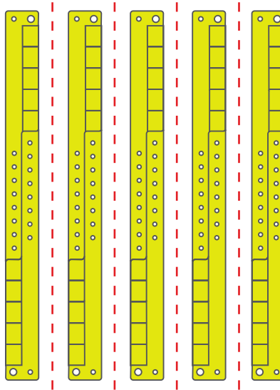
Rozdzielenie na 5 kpl. opasek
